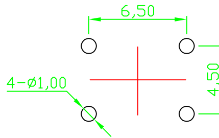
PCB. 焊接图
