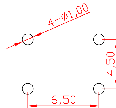
PCB. 焊接图
