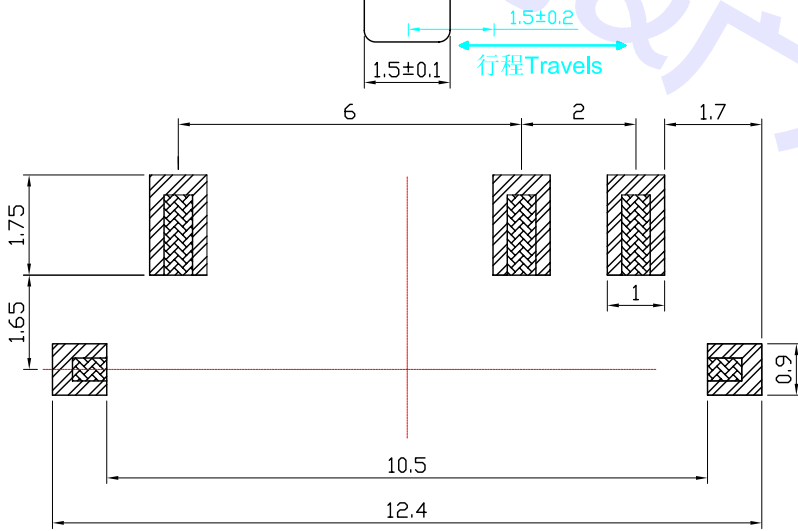
安装图 (PCB LAYOUT PLAN)
