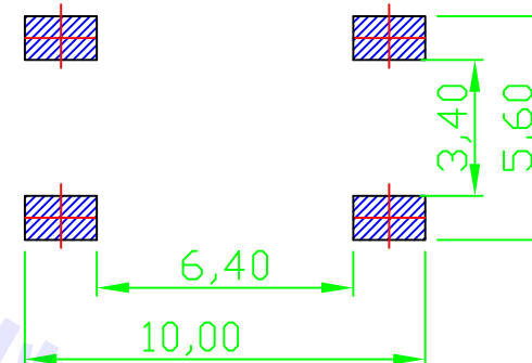
PCB. 焊接图
