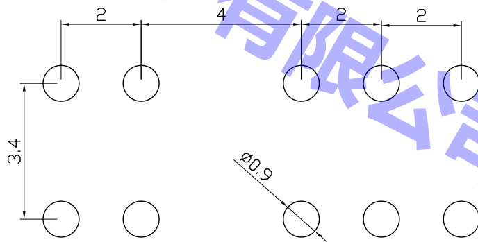
安装图 (PCB LAYOUT PLAN)
