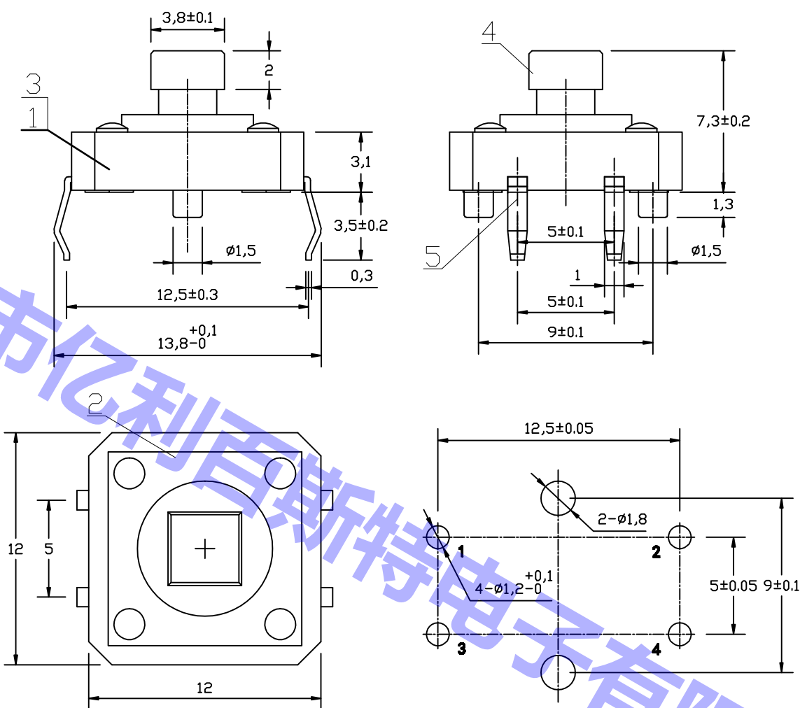
安装尺寸 (从焊锡面看)
