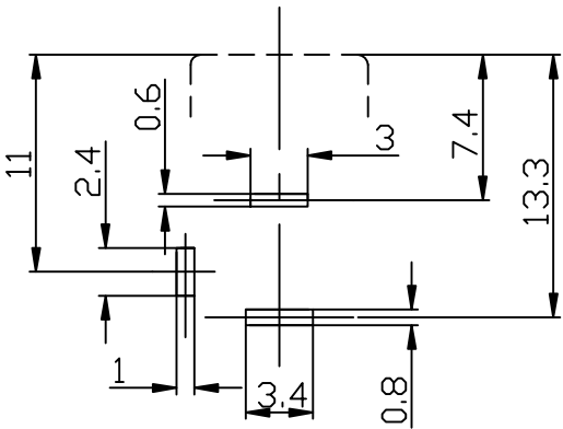
线路板开孔尺寸
