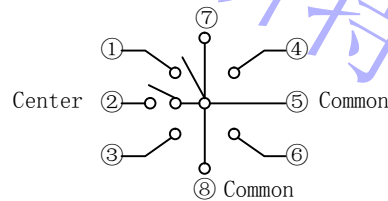
线路图
