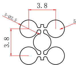
接触簧片
