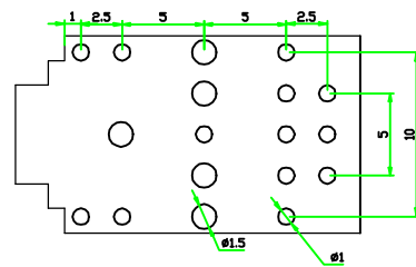
线路板安装图
