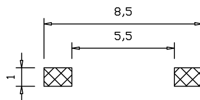
贴片尺寸 (从焊锡面看)
