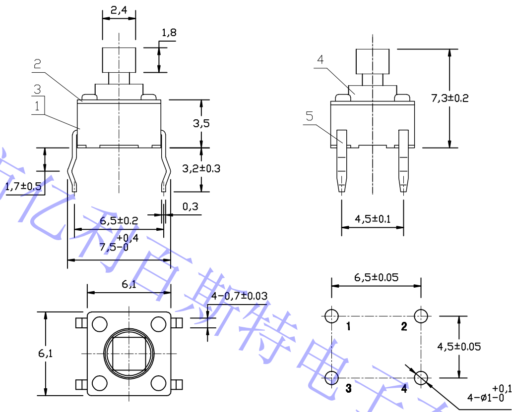
安装尺寸 (从焊锡面看)
